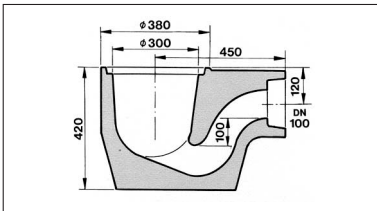
Bodenteil DN 100, mit Geruchverschluss, ohne Steckmuffe, DIN 1236-23
