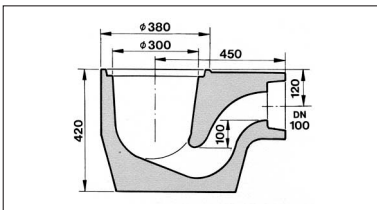
Bodenteil DN 100, mit Geruchverschluss, mit Steckmuffe für PVC-Kanalrohre
