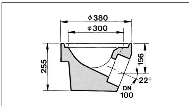
Bodenteil DN 100, ohne Geruchverschluss, ohne Steckmuffe für PVC-Kanalrohre
