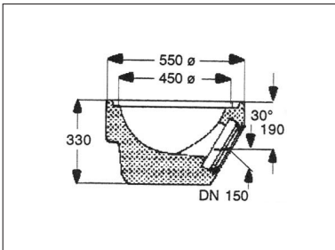
Bodenteil 1a, DIN 4052-1a mit Steckmuffe L für Steinzeugrohr DN 150
