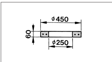
Auflagering, DIN 1236-28
