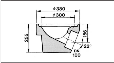
Bodenteil DN 100, ohne Geruchverschluss, ohne Steckmuffe, DIN 1236-21
