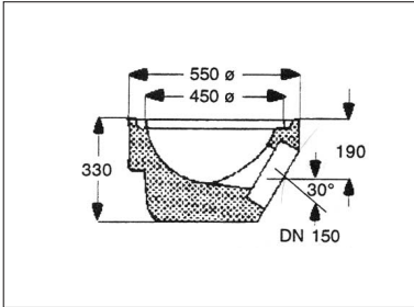
Bodenteil 1a, DIN 4052-1a ohne Steckmuffe DN 150
