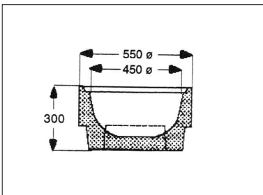
Bodenteil 2a, DIN 4052
