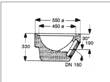
Bodenteil 1a, DIN 4052-1a mit Steckmuffe für PVC-Kanalrohre DN 150
