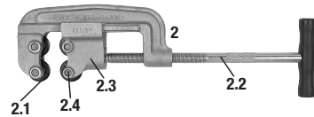
Vierrad-Rohrabschneider Art.-Nr. 715
