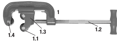
Dreirad-Rohrabschneider Art.-Nr. 715/1
