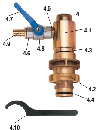
Aufschraubstück mit Spülhahn
